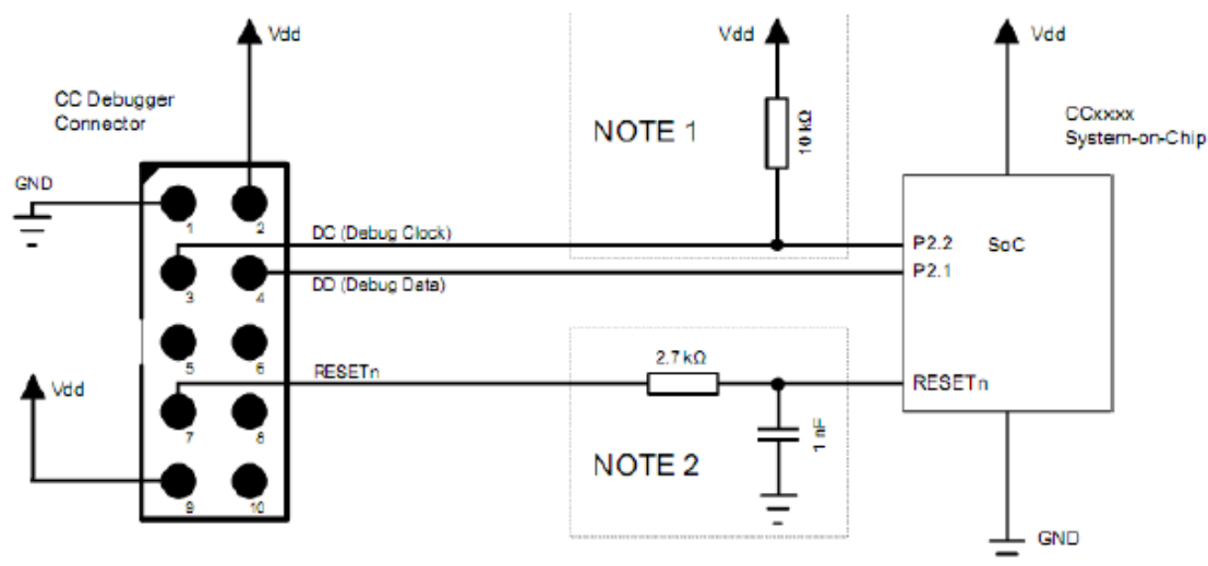
编程器和调试口连接图
