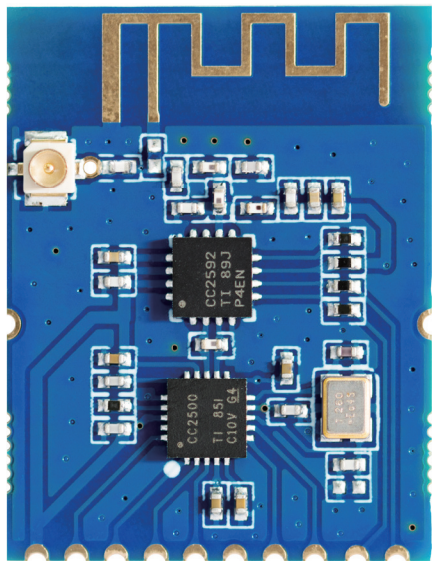
A款（外置天线）
