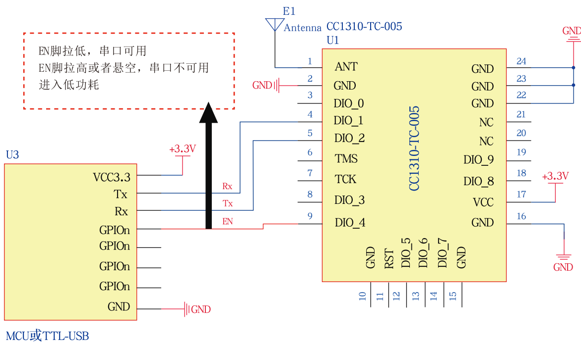
图 2 普通透传模块式
