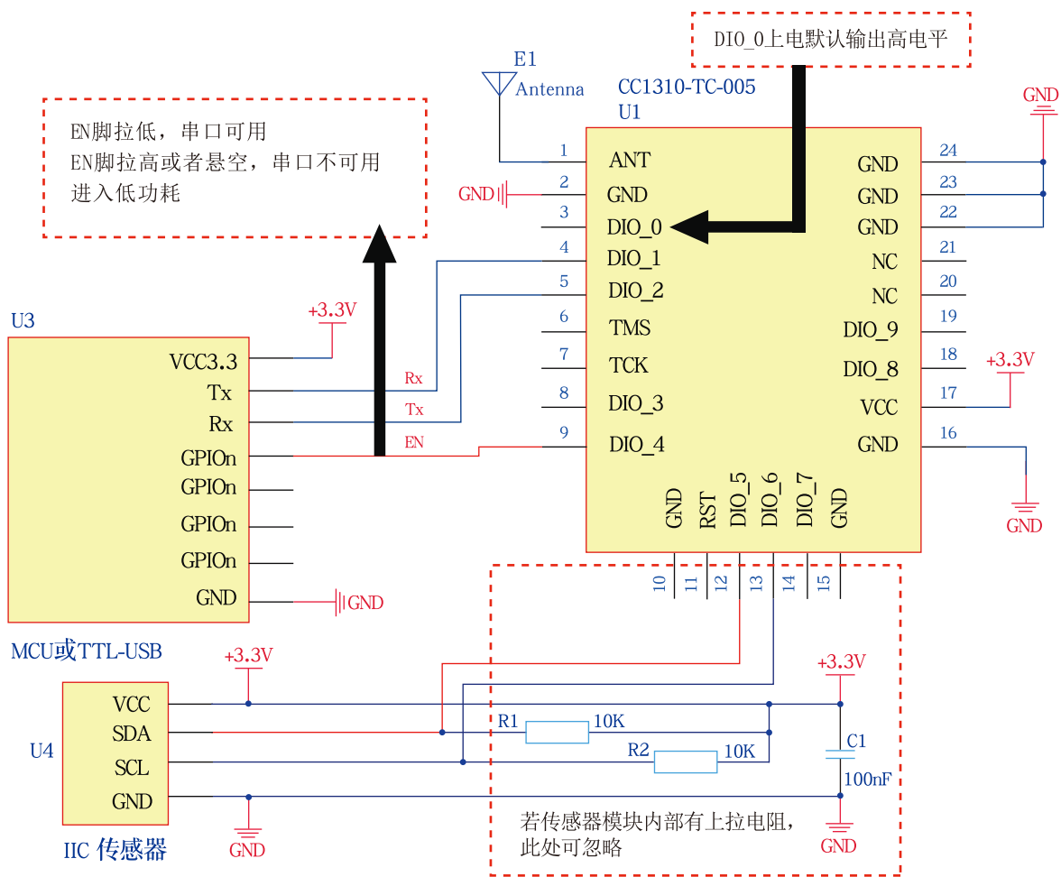
图 4 I2C传感器模式
