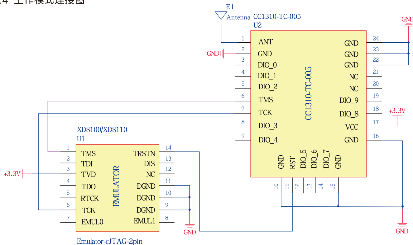
图 1 二次开发接线图
